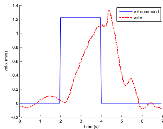
شکل ۱۱ - نتیجه آزمایش عملی کنترل کننده سرعت در راستای X با ضریب بهره ۱۰
