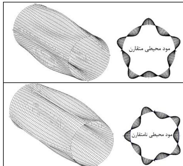
شکل 4- مودهای ارتعاشی به ازای n=5 و m=1
