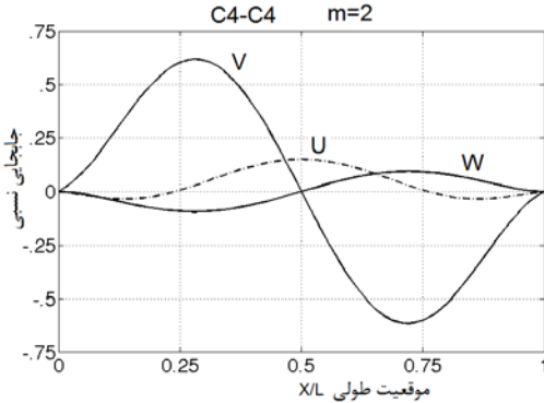
شکل 10- مودهای ارتعاشی تکیه گاه گیردار از نوع C4-C4
