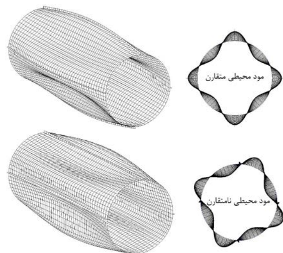
شکل 3- مودهای ارتعاشی به ازای n=4 و m=1
