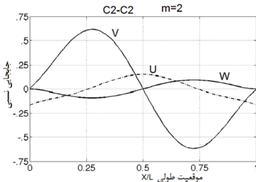
شکل 9- مودهای ارتعاشی تکیه گاه گیردار از نوع C2-C2
