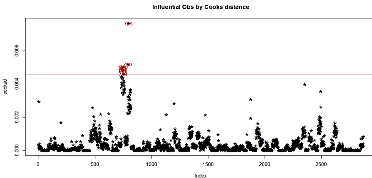
شکل ۲: بررسی مشاهدات پرت با رویکرد Cook's distance
