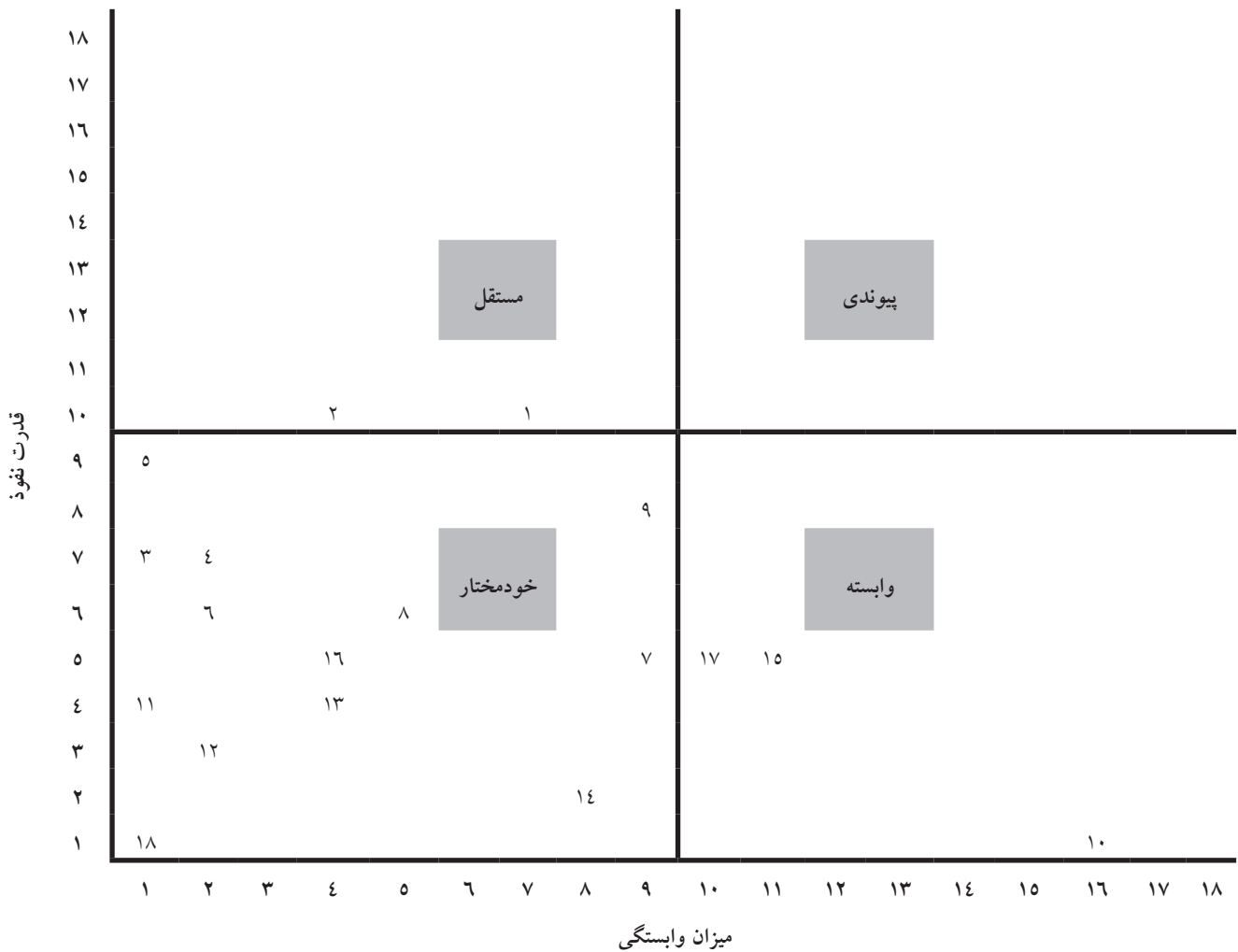
شکل ۲: تحلیل MICMAC
