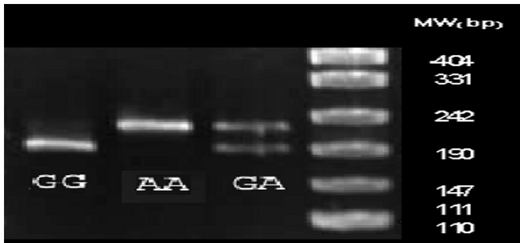
شکل ۲: پلی مورفیسم ژن IL 13 در جایگاه ۲۰۴۴+ بعد از هضم آنزیم NlaIV
