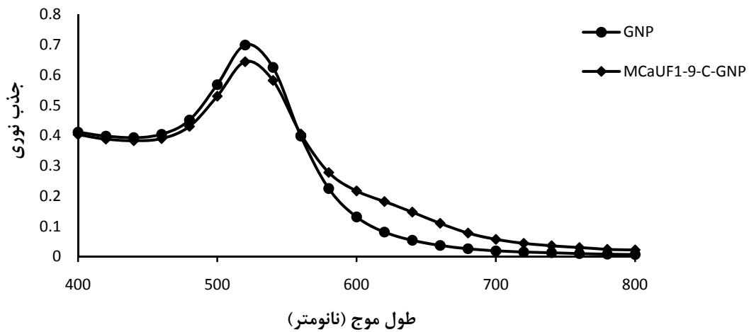
شکل ۱: طیف جذبی نانوذره طلا به تنهایی (GNP)، و نانوذره بعد از اتصال به پیپتید \text{MCAUF1-9-C} ( \text{MCAUF1-9-C-GNP} ، ۱۰۰ نانومولار)
