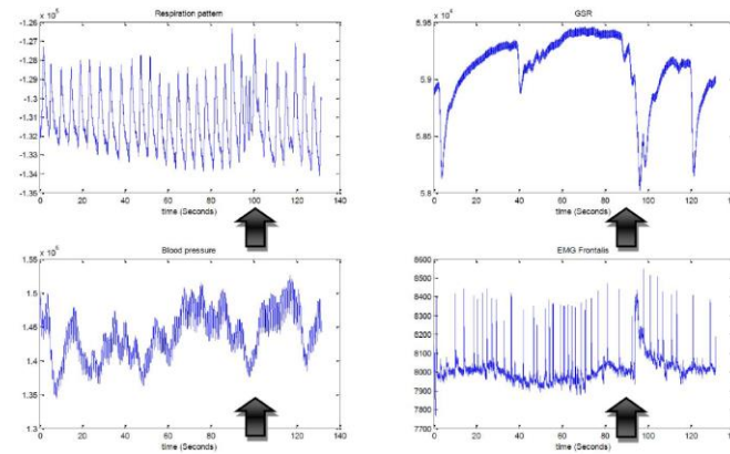
شکل ۴: پاسخ فیزیولوژیک دومین شرکت کننده به یک صحنه تعجب آور؛ الگوی تنفس (شکل بالا سمت چپ)، سیگنال GSR (شکل بالا سمت راست)، فشار خون (شکل پایین سمت چپ) و سیگنال EMG مربوط به پیشانی (شکل پایین سمت راست). لحظه ای که شرکت کننده دچار تعجب می شود با فلش در شکل ها نشان داده شده است [۱۸].
