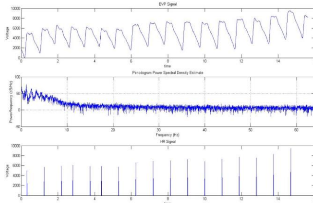
شکل ۹: نمونه‌ای از سیگنال BVP از نمونه شماره یک الف (سیگنال BVP) طیف فرکانسی سیگنال "الف" ج) سیگنال نرخ ضربان قلب (Heart Rate) استخراج شده از سیگنال "الف".
