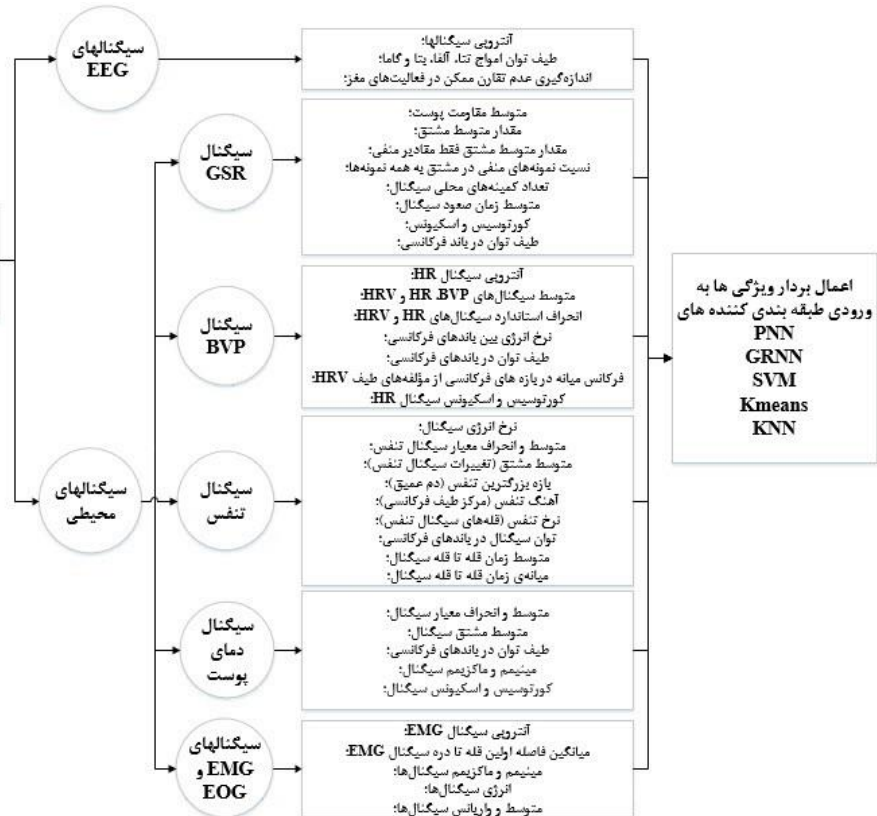
شکل ۶: بلوک دیاگرام مراحل انجام پژوهش
