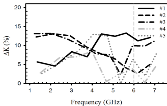
شکل ۱۴. اختلاف نتایج تحلیلی امپدانس برهمکنش مدل پیشنهادی به‌ازای m=-2:2 با نتایج شبیه‌سازی ماریپچ دوگانه
