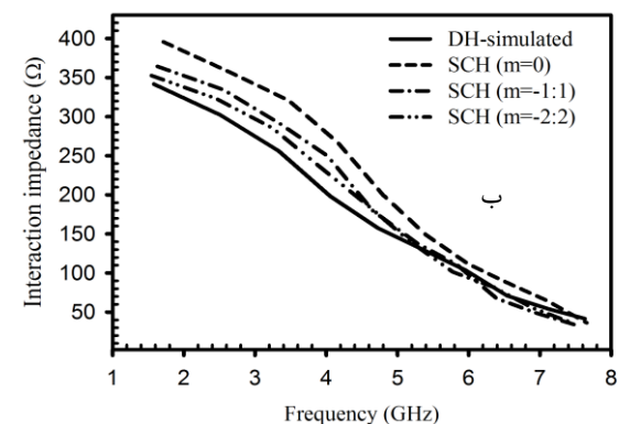
شکل ۱۳. نتایج تحلیلی امپدانس برهمکنش مدل ارائه‌شده به‌ازای مقادیر مختلفی از جملات m و مقایسه با نتایج شبیه‌سازی ماریپچ دوگانه به‌ازای a=2 mm, P=2 , الف- حالت چهارم با b=5/5 mm و ب- حالت پنجم با b=6 mm
