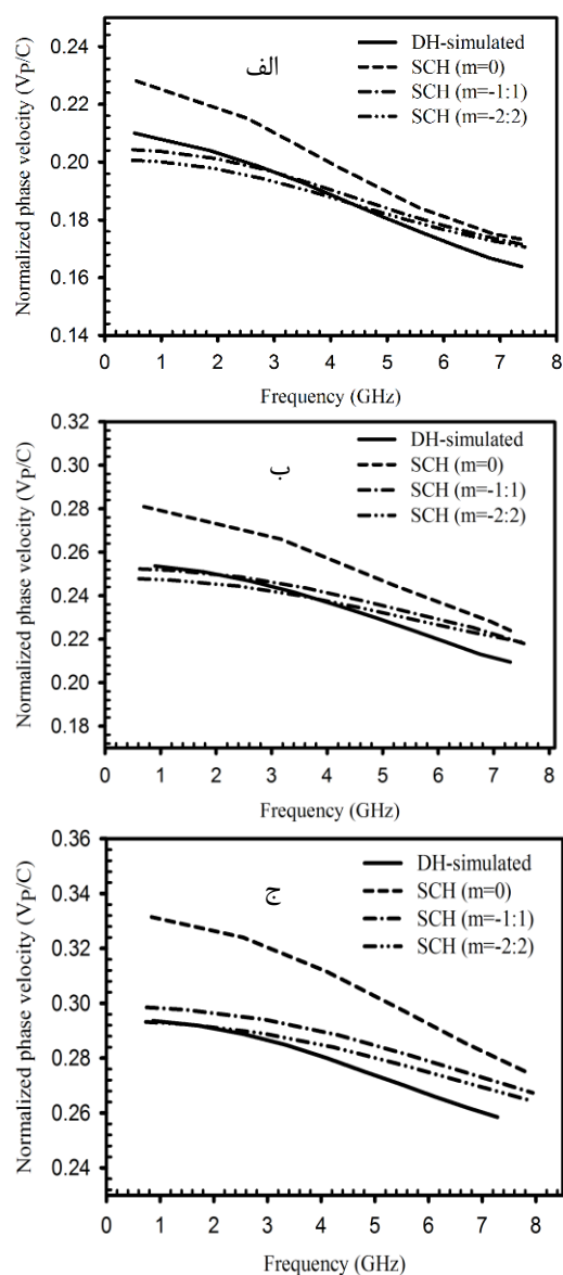
شکل ۹. نتایج تحلیلی سرعت فاز مدل ارائه‌شده به‌ازای مقادیر مختلفی از جملات m و مقایسه با نتایج شبیه‌سازی ماریپچ دوگانه به‌ازای a=2 mm، b=5 mm، الف-حالت اول با P=2 mm، ب- حالت دوم با P=5/5 mm و ج- حالت سوم P=3 mm
