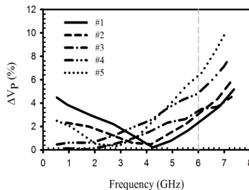
شکل ۱۱. اختلاف نتایج تحلیلی سرعت فاز مدل پیشنهادی به ازای m=-2:2 با نتایج شبیه سازی مارپیچ دوگانه
