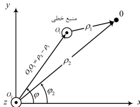
شکل ۸. موقعیت مکانی منبع جابه جا شده نسبت به مبدأ مختصات [۳۴]
