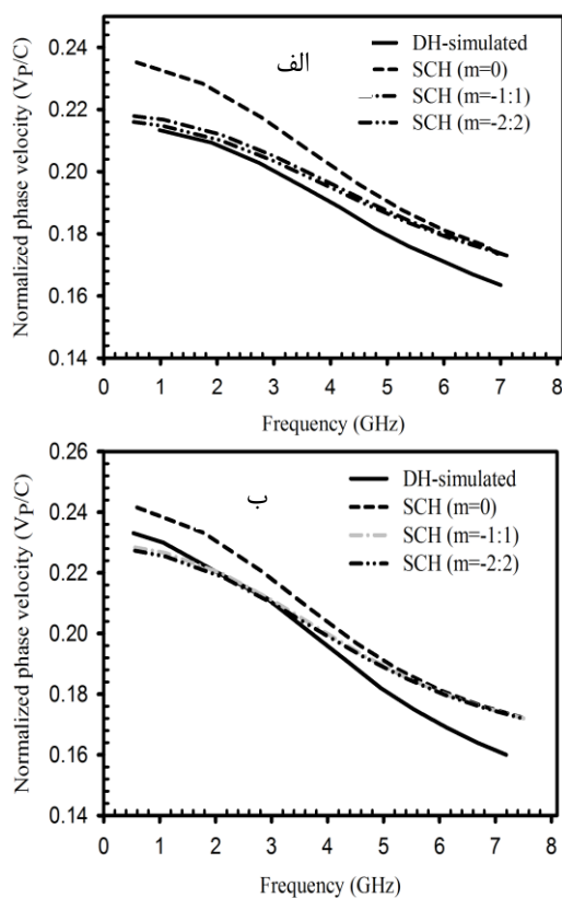
شکل ۱۰. نتایج تحلیلی سرعت فاز مدل ارائه‌شده به‌ازای مقادیر مختلفی از جملات m و مقایسه با نتایج شبیه‌سازی ماریپچ دوگانه به‌ازای a=2 mm، P=2 mm، الف- حالت چهارم b=5/5 mm و ب- حالت پنجم b=6 mm
