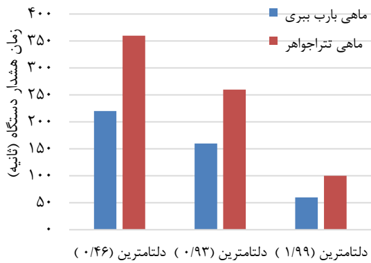
شکل ۱۲. مقایسه زمان هشدار دستگاه پس از ورود سم دلتامترین (گرم در لیتر) دلتامترین (۱/۹۹) دلتامترین (۰/۹۳) دلتامترین (۰/۴۶)
