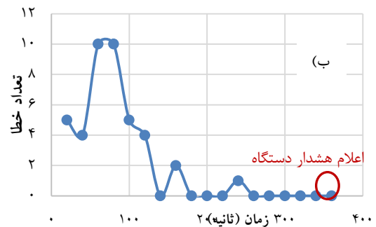
شکل ۹. عملکرد و خروجی دستگاه سمیت‌شناسی آب پس از ورود سم (علف‌کش دلتامترین با غلظت ۰/۴۶ گرم در لیتر) (الف ماهی بارب ببری ب) ماهی تترا جواهر
