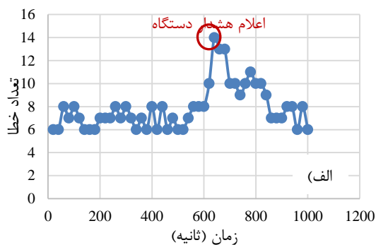
شکل ۵. عملکرد و خروجی دستگاه سمیت‌شناسی آب پس از ورود سم (علف‌کش توفوردی+ام‌سی‌پی‌آ با غلظت ۱۷/۴ گرم در لیتر) (الف) ماهی بارب ببری (ب) ماهی تترا جواهر
