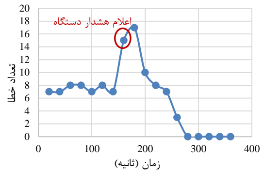
شکل ۹. عملکرد و خروجی دستگاه سمیت‌شناسی آب پس از ورود سم (علف‌کش دلتامترین با غلظت ۰/۴۶ گرم در لیتر) (الف ماهی بارب ببری ب) ماهی تترا جواهر
