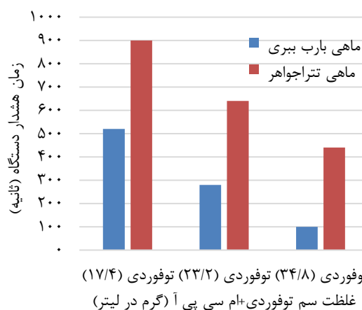
شکل ۸. مقایسه زمان هشدار دستگاه پس از ورود سم توفوردی+ام‌سی‌پی‌آ
