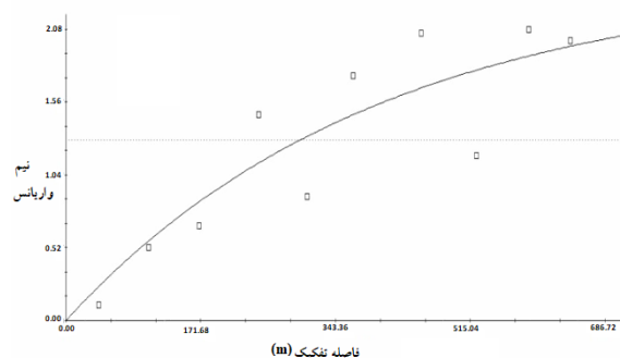
شکل ۸- نمودار واریوگرام داده‌ها و در موقعیت‌های مکانی مشاهده‌ای
