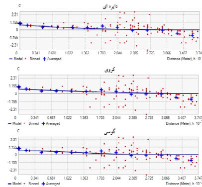
شکل ۱۷- نیم پراش نگار (دایره‌ای، کروی، گاوسی) کمینه انرژی تابشی ادارات در مدل کریجینگ معمولی جولای
