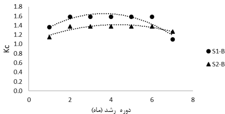
شکل ۷- ضریب گیاهی سالیکورنیا - بیگلووی در دو شوری متفاوت در فصل رشد (علائم مشابه شکل ۶)
