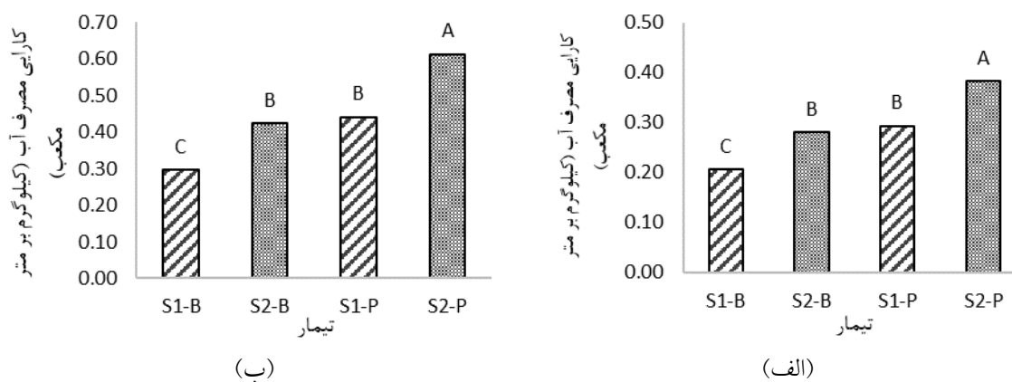
شکل ۹- کارایی مصرف آب در تیمارهای مختلف (الف) بر اساس آب مصرفی و (ب) بر اساس تبخیر و تعرق (علائم مشابه شکل ۶)
