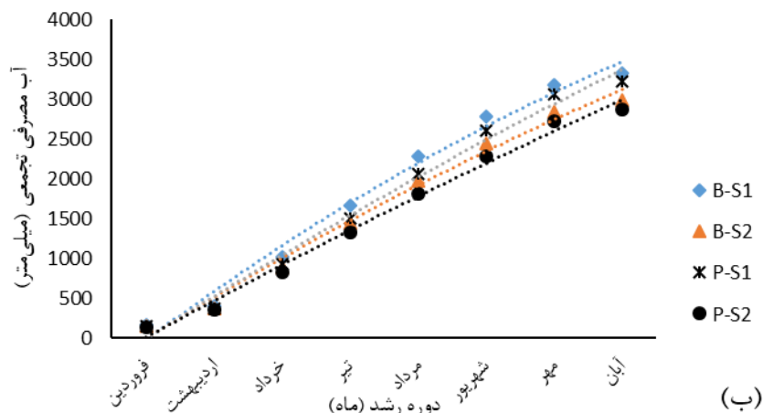
شکل ۶- میزان تبخیر و تعرق (الف) و آب مصرفی (ب) تجمعی دو گونه سالیکورنیا در تیمارهای مختلف (علائم B-S1 و B-S2 به ترتیب بیانگر گونه بیگلووی در سطح شوری یک و دو و علائم P-S1 و P-S2 به ترتیب بیانگر گونه پرسیکا سطح شوری یک و دو می باشند)
