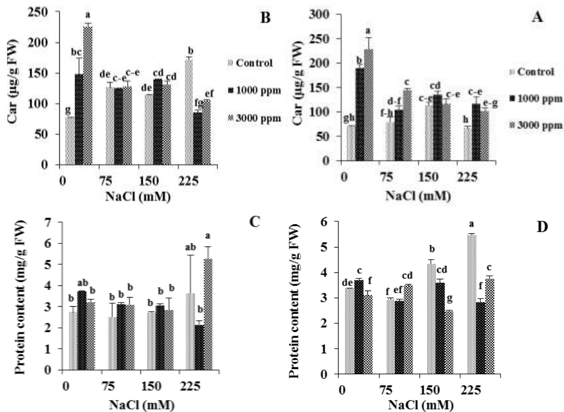
شکل ۲- اثر متقابل نانوذره اکسید روی و شوری کلرید سدیم بر میزان [۱- کاروتنوئید (میکروگرم/گرم وزن تر در رقم اردستانی (A)، رقم مشدی (B) و میزان پروتئین کل (میلی گرم/گرم وزن تر) در رقم اردستانی (C)، رقم مشدی (D)] گیاه شنبليله. میانگین داده‌ها حاصل از سه تکرار و مقایسه میانگین‌ها بر اساس آزمون توکی می‌باشد ( P \leq 0.05 ).
