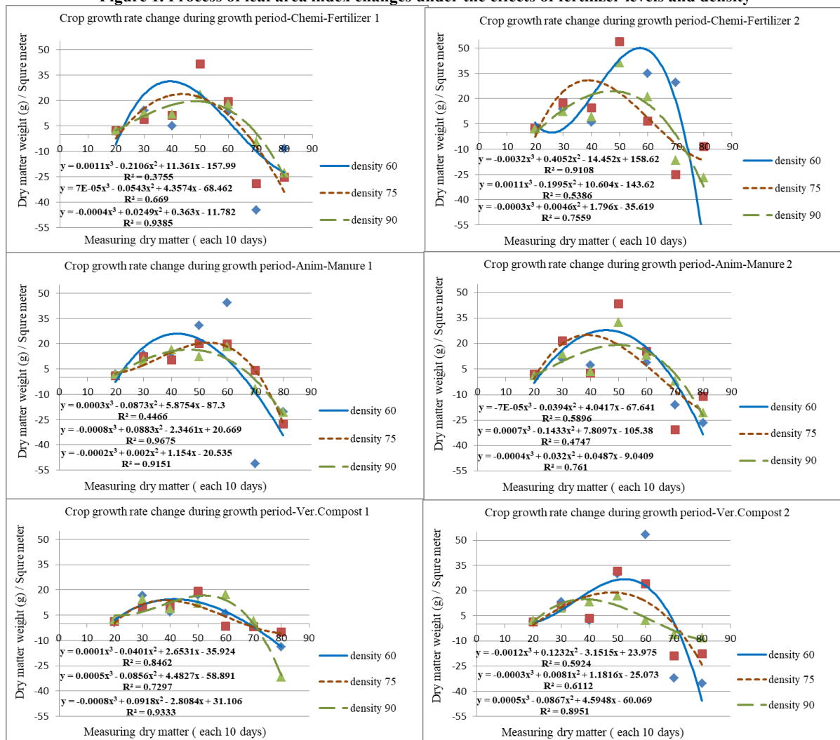
شکل ۲. روند تغییرات سرعت رشد محصول (CGR) تحت تاثیر سطوح کود و تراکم
