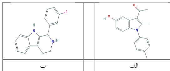
شکل ۷) ساختار مولکولی دو ترکیب ایندولی شناسایی شده در عصاره متانول-کلروفرمی جلبک سارگاسوم بوویانوم. ساختار پیریدو (ب) [۳-۴-ب] ایندول اتانون (الف)؛ ۱- [۵-هیدروکسی-۲-متیل-۱-(پی-تولیل)-۳-ایندول] اتانون (ب).
