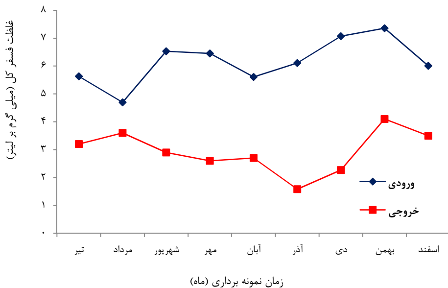
نمودار ۳- روند تغییرات فسفات کل در تصفیه خانه فاضلاب شهر یزد (در طی ماه‌های مختلف نمونه برداری سال ۱۳۹۷)
