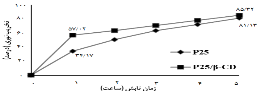
شکل ۷. تخریب نوری ۴۲-دی کلروفنوکیسی استیک اسید (۲۰ mg/L) با نانو نور کاتالیزگر P25 (۵۰ mg) و P25/β-CD (۵۵ mg) در راکتور نوری با جریان ناپیوسته (منبع تابش: LED با توان ۲۰ وات، طول موج ۴۰۰ نانومتر و شدت جذب (۱۰۰ mW/cm
