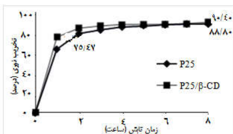
شکل ۸. تخریب نوری ۴۰۲-دی کلروفنوکی استیک اسید (۲۰ mg/L) با نانو کاتالیزگر P25 (۵۰۰ mg) و P25/β-CD (۵۵۰ mg) در راکتور نوری با جریان پیوسته (منبع تابش: مجموع LED ها با توان ۱۰۰ وات، طول موج ۳۶۵ نانومتر و شدت جذب ۱۰۰ mW/cm) در راکتور نوری با جریان پیوسته
