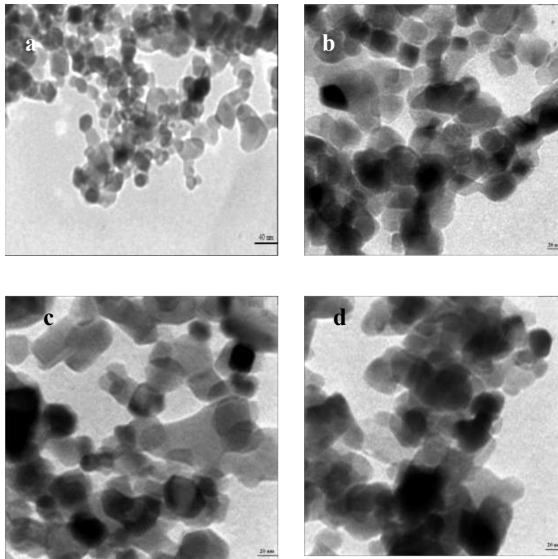
شکل ۴. تصاویر میکروسکوپ الکترونی نانونور کاتالیز گر P25 (a)، P25/ \beta -CD (b)، P25 (c) (بعد از سیکل ۵) و \beta -P25/CD (بعد از سیکل ۵)
