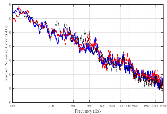
شکل ۹- نمودار سطح فشار صوت برای سه موقعیت مکانی مختلف در اتاق پربازتاب
