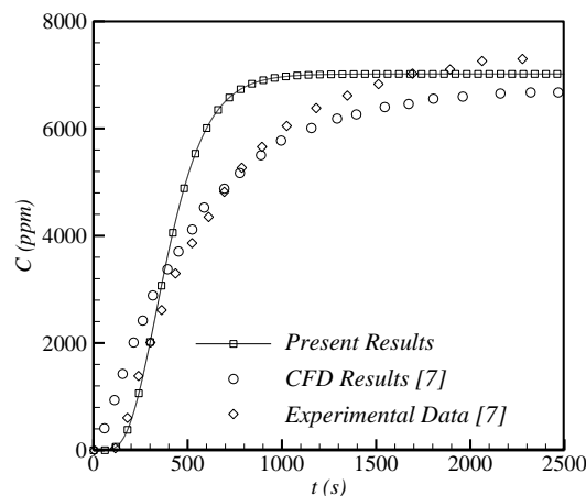
شکل ۷- مقایسه نتایج تغییرات غلظت- سنسور شماره ۲
