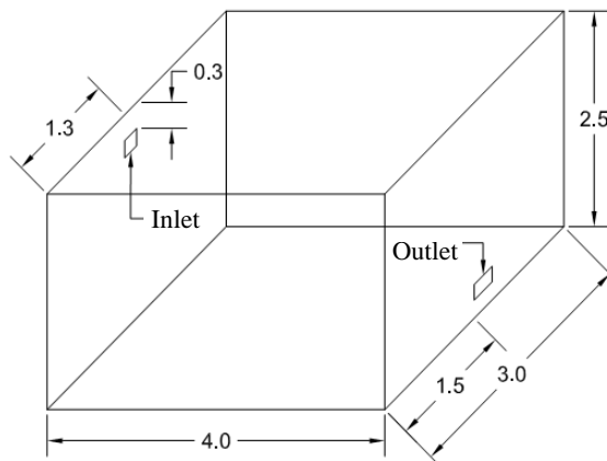
شکل ۲- مشخصات اتاق مورد استفاده جهت شبیه‌سازی [۷] (ابعاد بر حسب متر)
