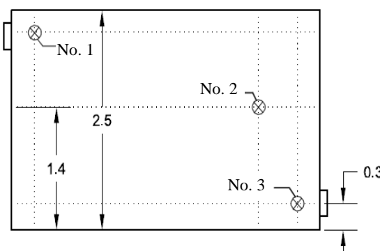
شکل ۳- محل سنسورهای سنجش غلظت آلودگی در اتاق [۷] (ابعاد بر حسب متر)
