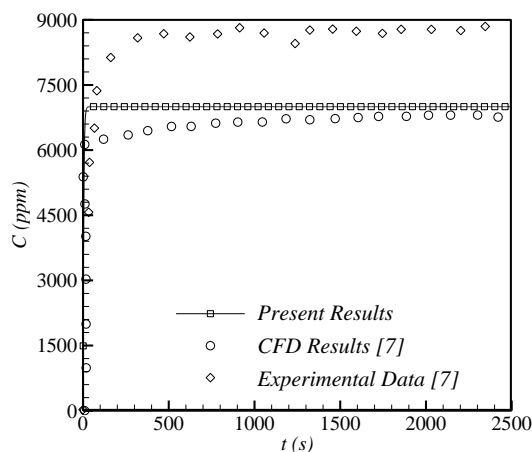
شکل ۶- مقایسه نتایج تغییرات غلظت- سنسور شماره ۱
