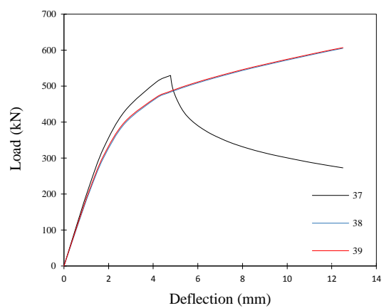
شکل ۱۸- نمودارهای بار-تغییر مکان نمونه‌های ۳۷ تا ۳۹
