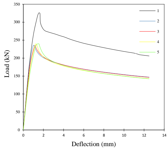
شکل ۶- نمودارهای بار-تغییرمکان نمونه‌های ۱ تا ۵
