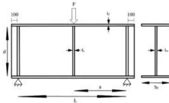
شکل ۱- هندسه و طرح بارگذاری نمونه‌ی مورد آزمایش
