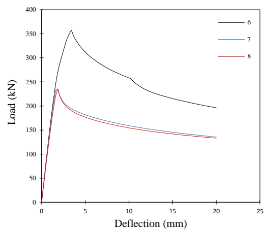
شکل ۷- نمودارهای بار-تغییرمکان نمونه‌های ۶ تا ۸
