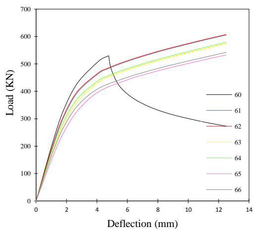
شکل ۲۳- نمودارهای بار-تغییرمکان نمونه‌های ۶۰ تا ۶۶
