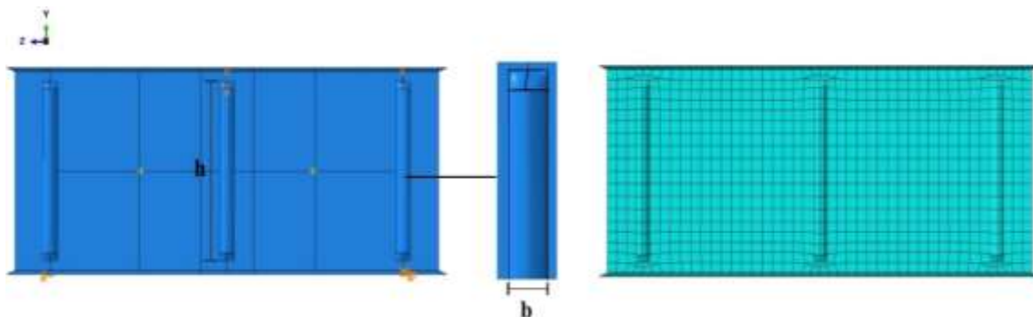
شکل ۵- تیرورق با جان موج دار محلی (پرس)
