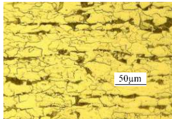
شکل ۴- فلز پایه
