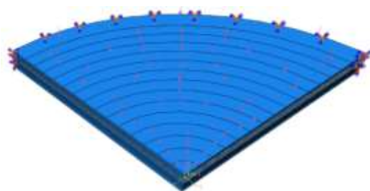
شکل ۱۱- نحوه اعمال بارگذاری انفجاری و شرایط مرزی
