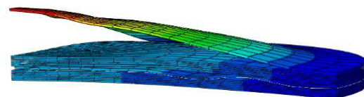
شکل ۲۰- شبیه‌سازی نمونه ۳
