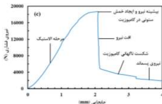
شکل ۶- نمودار نیرو-جابجایی برای، (a) حالت ۱ شکست (نمونه gjzjg)، (b) حالت ۲ شکست (نمونه jzjzjg)، (c) حالت ۳ شکست (نمونه gjzjg)
