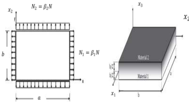
شکل ۱- نمایش یک نانو ورق مستطیلی هدفمند نسبتاً ضخیم با دستگاه مختصات در نظر گرفته شده در لایه میانی
