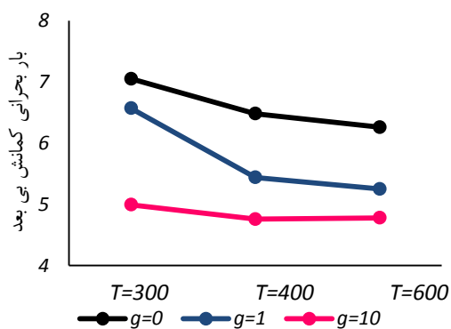
شکل ۲- تغییر بار بحرانی کمانش بی بعد \bar{N}_{cr} = \frac{N_{cr} a^2}{E_m h^3} نسبت به دما با بکارگیری تئوری تغییر شکل برشی نمایی تحت شرط مرزی SCSC
