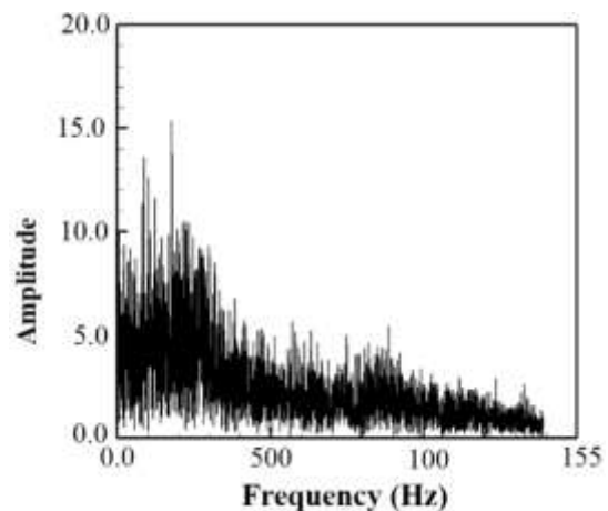
شکل ۱۹- نمودار پاسخ فرکانسی نسبت فشار حسگر T21 در نسبت انسداد ۵۵٪ با استفاده از روش FFT ۲
