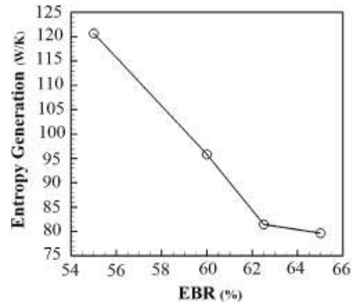
شکل ۱۱- نمودار تولید آنتروپی بر حسب نسبت انسداد
