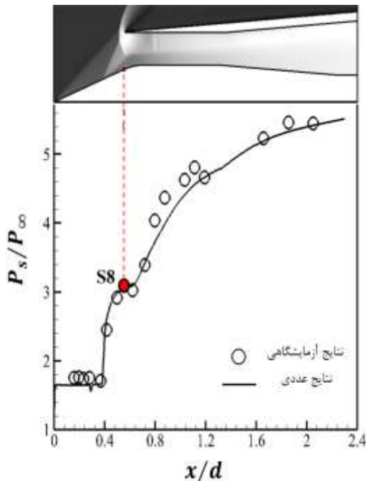
شکل ۱۶- نسبت فشار استاتیکی روی اسپایک در حالت
