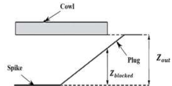
شکل ۶- پارامترهای مربوط به نسبت انسداد خروجی
