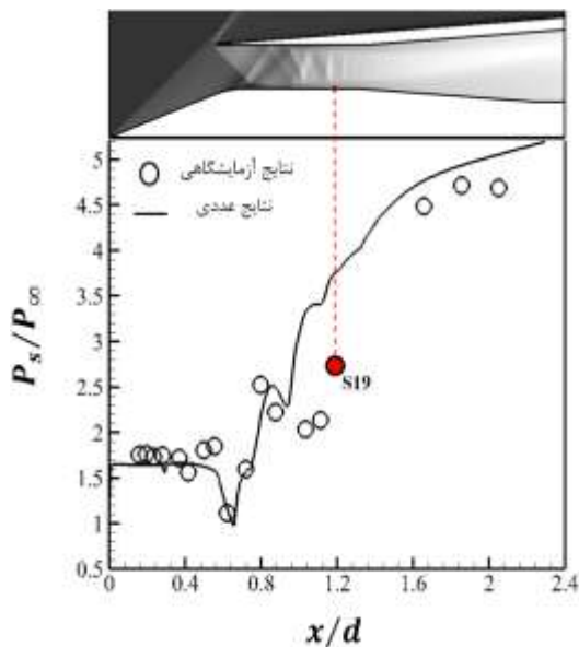
شکل ۱۴- نسبت فشار استاتیکی روی اسپایک در حالت عددی و تجربی در نسبت انسداد ۶۰٪
