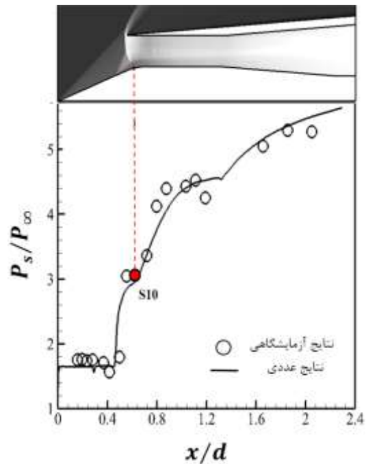
شکل ۱۵- نسبت فشار استاتیکی روی اسپایک در حالت عددی و تجربی در نسبت انسداد ۰.۶۲/۵
