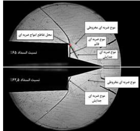
شکل ۱۷- مقایسه زاویه موج ضربه‌ای جدایش در دو نسبت انسداد ۶۵٪ و ۶۲.۵٪
