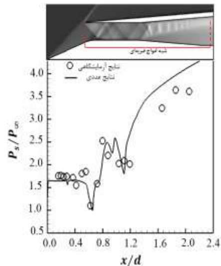
شکل ۹- مقایسه نسبت فشار استاتیکی روی اسپایک حاصل از نتایج عددی و تجربی در نسبت انسداد ۵۵٪
