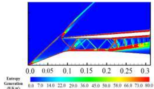
شکل ۱۲- کانتور تولید آنتروپی در نسبت انسداد ۵۵٪
