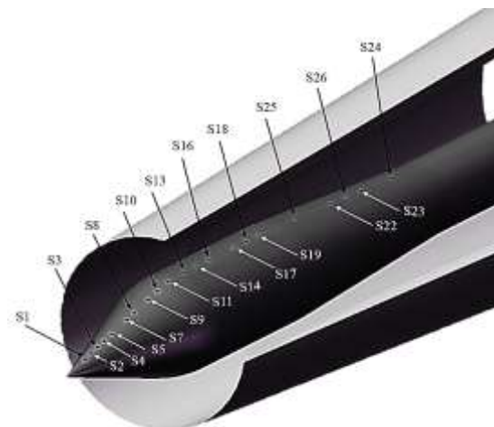
شکل ۵- نام و مکان قرارگیری حسگرهای فشار استاتیک
