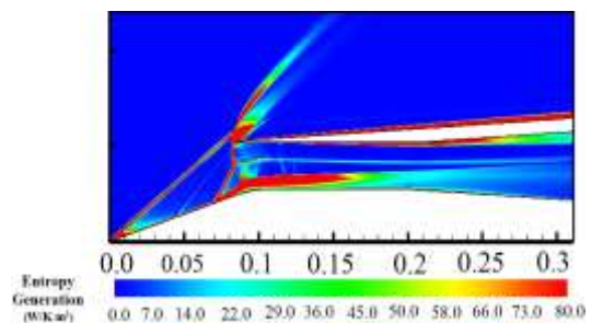
شکل ۱۳- کانتور تولید آنتروپی در نسبت انسداد ۶۲/۵٪
