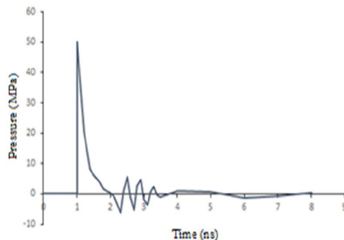
شکل ۶- بار انفجار [۱۷]
