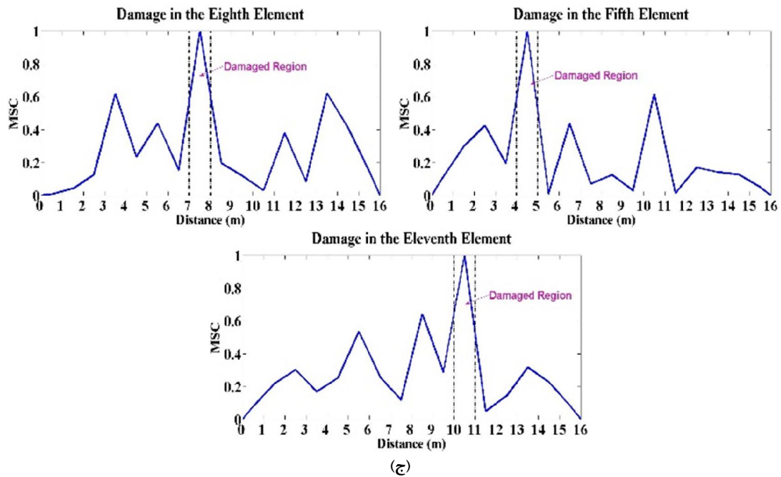
شکل ۷- شناسایی مکان ترک با شدت ۲۰٪ در المان‌های ۵، ۸ و ۱۱ با در نظر گرفتن الف) ۵٪، ب) ۱۰٪ و ج) ۱۵٪ نویز در اندازه‌گیری
