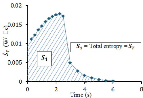
شکل ۱۱- نرخ انتروپی و انتروپی کل در فرایند لیزر فرمینگ در شرایطی که توان، سرعت اسکن، قطر پرتو و ضخامت ورق به ترتیب برابر با ۱۱۰۰ وات، ۳۰ میلی متر بر ثانیه، ۴ و ۲ میلی متر می باشد
