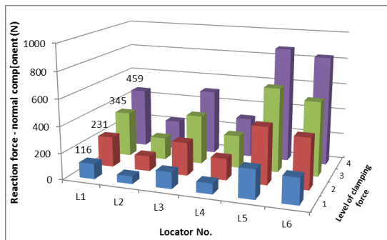
شکل ۵- مطالعه تأثیر اندازه نیروهای بست بر روی مؤلفه عمودی نیروی عکس‌العمل بدست آمده از شبیه‌سازی (ضریب اصطکاک: ۰/۳)
