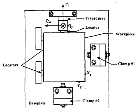
شکل ۲- مدل استفاده شده در [۲۵] به عنوان مطالعه موردی همراه با سیستم جاسازی و بست
