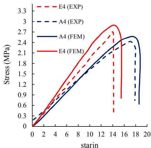
شکل ۷- نمودار تنش-کرنش آزمایش تک لبه برشی نمونه‌های E4 و A4 با نوع چسب متفاوت
