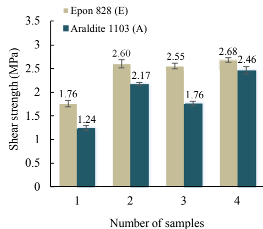
شکل ۴- تاثیر نوع چسب، ناحیه هم پوشانی و اصلاح سطحی بر استحکام برشی ساندویچ پنل‌ها
