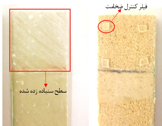
شکل ۱- آماده سازی سطح کامپوزیت و فوم PVC: الف) سطح کامپوزیت پلیمری اصلاح شده به روش سنباده‌زنی و ب) فیلرهای نصب شده برای کنترل ضخامت
