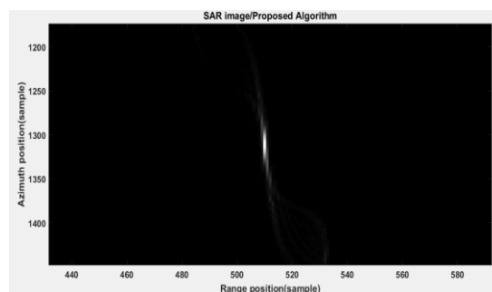
شکل (۱۵): تصویر سار با زاویه کجی ۲۰° (الگوریتم پیشنهادی)
