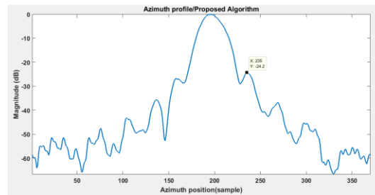
شکل (۱۰): پروفایل سمت هدف با زاویه کجی ۳° (الگوریتم پیشنهادی)
