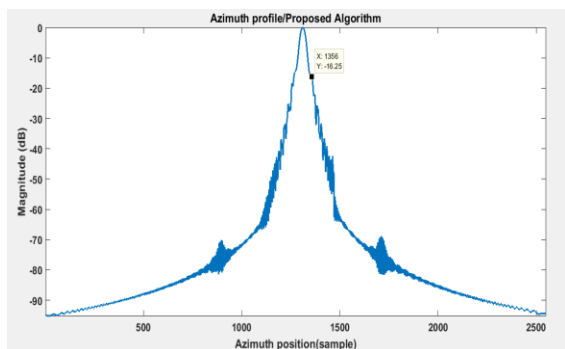
شکل (۱۱): پروفایل سمت هدف با زاویه کجی ۲۰° (الگوریتم پیشنهادی)
