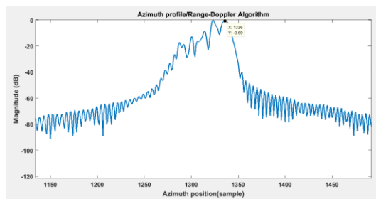
شکل (۱۴): بزرگنمایی شده شکل (۱۲)
