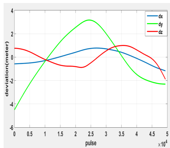
شکل (۱۷): انحرافات حرکتی پرنده در هر یک از راستاهای حرکت (z و y ,x)
