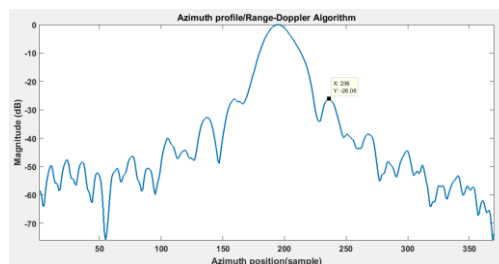
شکل (۹): پروفایل سمت هدف با زاویه کجی ۳° (الگوریتم برد-داپلر)
