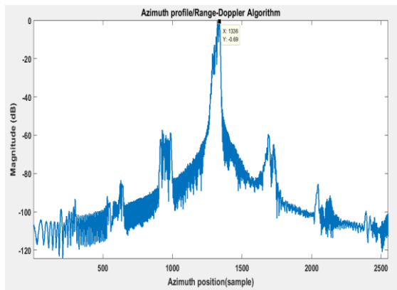
شکل (۱۲): پروفایل سمت هدف با زاویه کجی ۲۰° (الگوریتم برد-داپلر) جهت مقایسه بهتر شکل‌های (۱۱-۱۲)، بزرگنمایی پروفایل سمت هدف در شکل‌های (۱۳-۱۴) رسم گردیده است.
