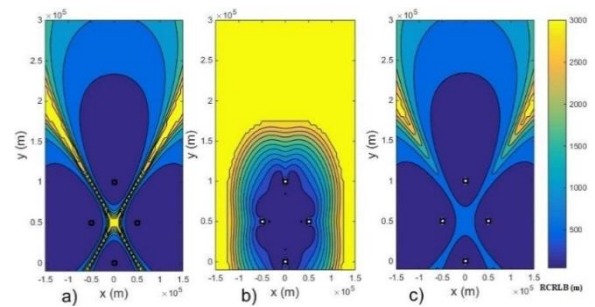
شکل (۶): RCRLB مکان‌یابی در محدوده X و Y برای اندازه‌گیری‌های TDOA و AOA زاویه سمت و ارتفاع با انحراف معیار خطای اندازه‌گیری به ترتیب برابر ۱۰۰ ns و ۱ deg و ۳ deg با ۳ فرستنده و ۴ گیرنده در فاصله دور برای (a) تنها TDOA، (b) تنها AOA و (c) AOA و TDOA ترکیبی.
