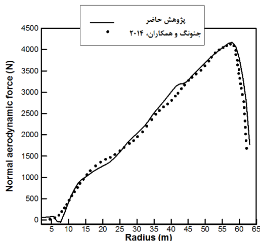
شکل (۴): مقایسه توزیع نیروی محوری در طول پره
