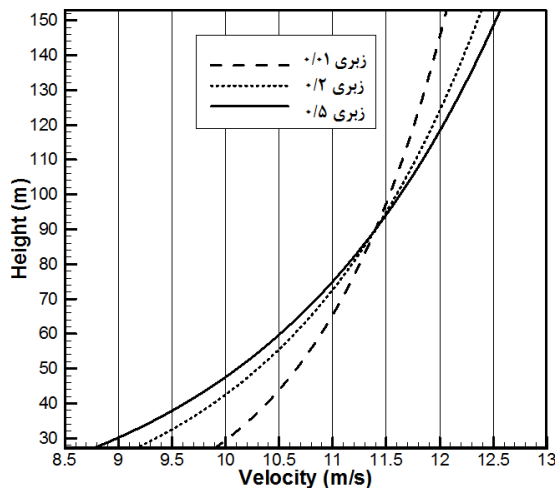
شکل (۱۱): سرعت جریان در ارتفاع روتور نسبت به زبری سطح
