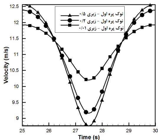
شکل (۱۳): سرعت باد در نوک پره حین دوران در زبری‌های مختلف
