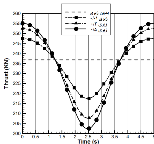
شکل (۱۹): تراست پره اول نسبت به زبری سطح
