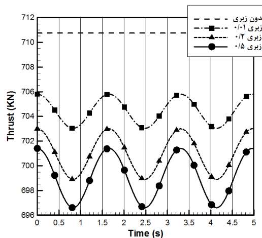
شکل (۲۰): تراست روتور نسبت به زبری سطح
