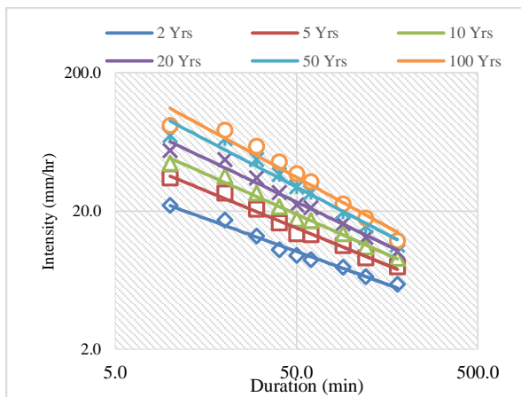
Fig. 6- IDF Curves for wet scenario شکل ۶- منحنی شدت مدت فراوانی تحت سناریو مرطوب
