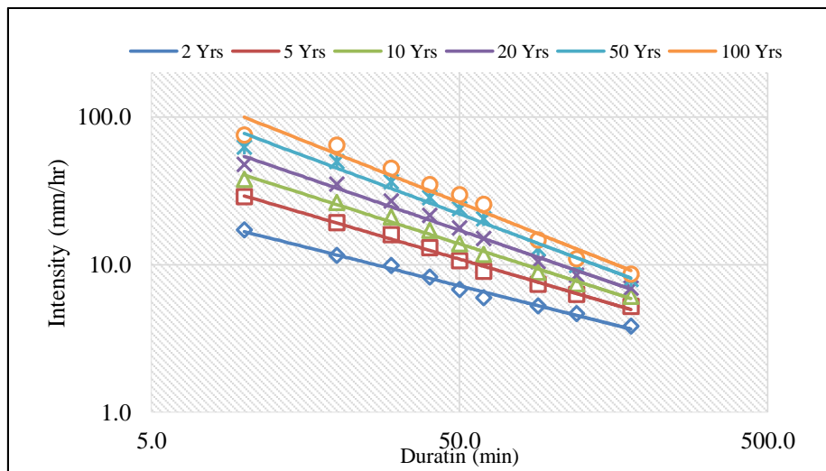
Fig. 4- IDF curves for base period شکل ۴- منحنی شدت مدت فراوانی داده‌های پایه
