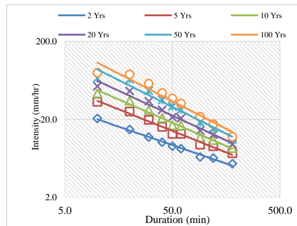
Fig. 5- IDF curves for historical scenario شکل ۵- منحنی شدت مدت فراوانی تحت سناریو تاریخی
