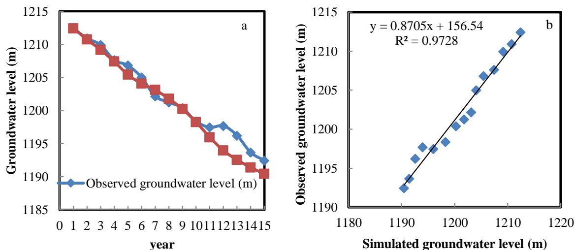
Fig. 6- a) The observed and simulated unit hydrograph of groundwater level and b) The linear regression between observed and simulated unit hydrograph of groundwater level during 15 years شکل ۶- (a) هیدروگراف واحد سطح ایستابی مشاهده شده و شبیه‌سازی شده با استفاده از مدل پویایی سیستم و (b) رگرسیون خطی بین هیدروگراف شبیه‌سازی شده و مشاهده شده در طول ۱۵ سال
