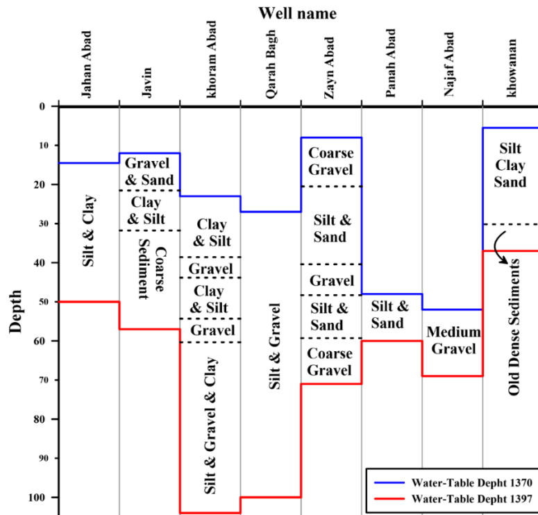
Fig. 15- Well logging in Water-level decline depth in the period of 1991-2018 شکل ۱۵- لایه بندی خاک در محدوده عمق افت آبخوان بین سالهای ۱۳۷۰ تا ۱۳۹۷
