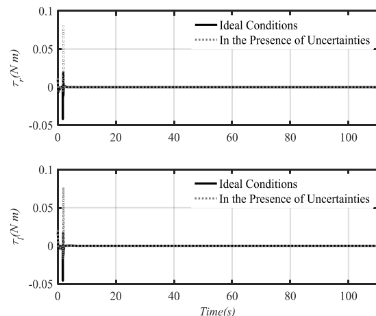
شکل (۱۴): سیگنال های کنترل در شرایط ایده آل و نامعینی پارامتری.
