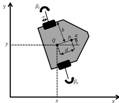
شکل (۱): ربات پایه متحرک چرخ‌دار.
