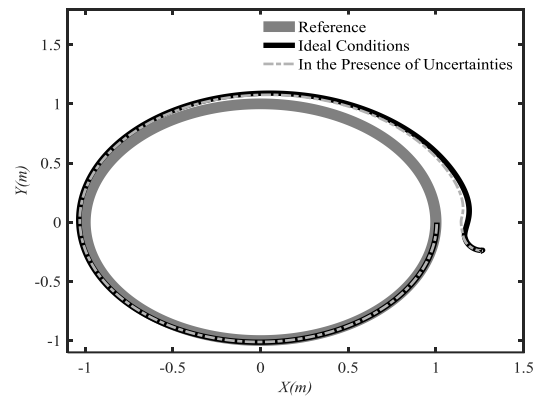
شکل (۱۲): مسیر ربات در شرایط ایده آل و نامعینی پارامتری
