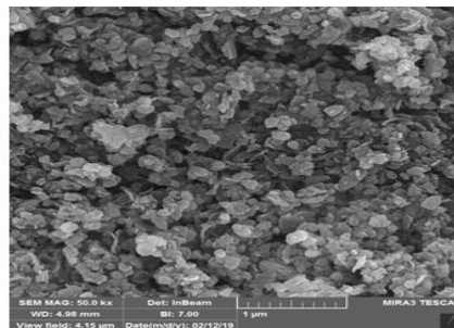
شکل شماره ۱. تصاویر میکروسکوپی (FESEM) نانوذرات اکسیدروی سنتز شده توسط مواد درون سلولی مخمر
