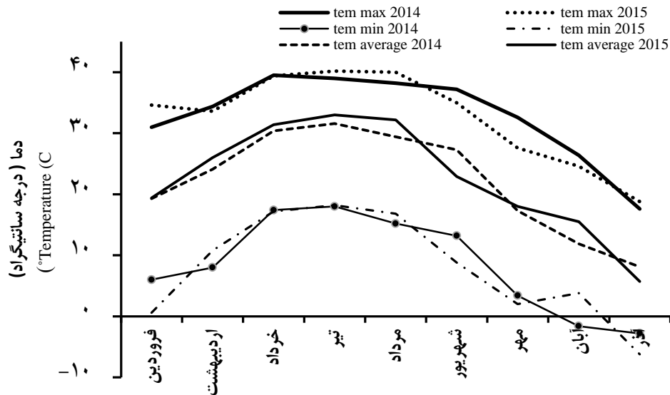
شکل ۱- کمینه، بیشینه و متوسط دما در دوره رشد پنبه در سال‌های ۱۳۹۳ و ۱۳۹۴
