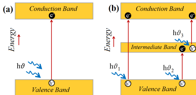
شکل ۲. گذارهای محتمل در (الف) ساختارهای نیم‌رسانای معمولی، (ب) ساختارهای نیم‌رسانای دارای باند میانی.
