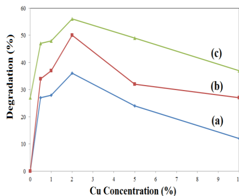
شکل ۸. تخریب MB با فیلم‌های نازک ZnS حاوی غلظت‌های مختلف Cu برای زمان‌های واکنش مختلف، (الف) ۳۰ دقیقه، (ب) ۱۲۰ دقیقه، (ج) ۳۶۰ دقیقه.
