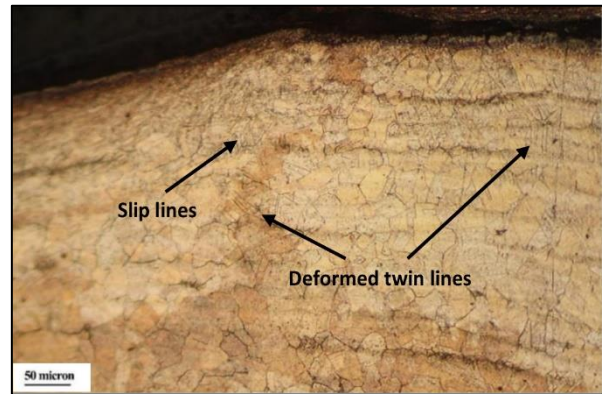
شکل ۲. شکل متالوگرافی نمونه S10-16 نشان دهنده ریزساختار با دانه های باز تبلور یافته و دارای دوقلوبی های تغییر شکل یافته و خطوط لغزش.
