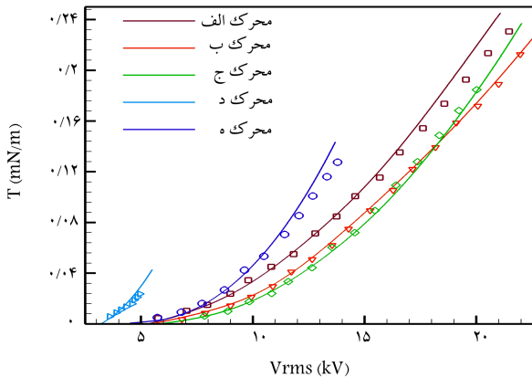
شکل ۲. اعتبارسنجی نیروی پیشران تولیدی در مقایسه با تجربی [۲۲] (خطوط: نتایج مطالعه حاضر، نشانه‌ها: نتایج تجربی).
