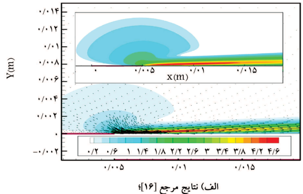
شکل ۷. مقایسه‌ی توزیع غلظت پلاسمای تولیدی.
