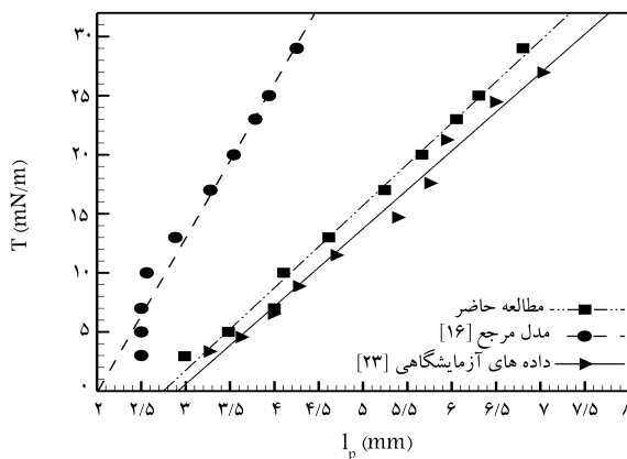
شکل ۳. اعتبارسنجی معادله‌ی طول پلازما در مدل پیشنهادی و مقایسه‌ی آن با نتایج تجربی [۲۳] و الگوی مرجع [۱۶].
