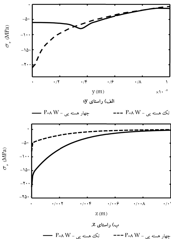
شکل ۱۳. مقایسه‌ی توزیع تنش ( \sigma_r ) در حالت چهارهسته‌یی و تک‌هسته‌یی.
