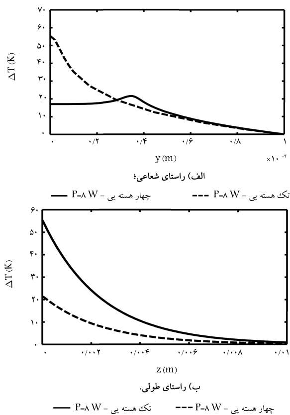
شکل ۱۴. مقایسه‌ی تغییرات دما در حالت چهارهسته‌یی و تک‌هسته‌یی.
