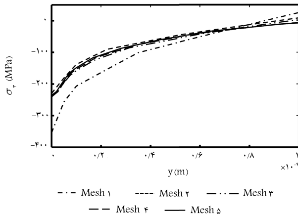
شکل ۵. توزیع بیشینه تنش ( \sigma_r ) در راستای شعاعی، برای توان ورودی ۹ وات در مش‌های متفاوت.
