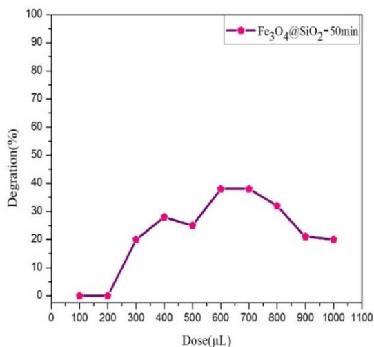
شکل 16. درصد تخریب دیازینون در حضور Fe_3O_4@SiO_2 .
