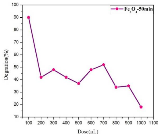
شکل 13. درصد تخریب دیازینون در حضور نانوذرات Fe_3O_4 .
