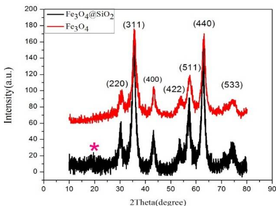
شکل 7. الگوی XRD نانو ذرات \text{Fe}_3\text{O}_4 و نانو ذرات هسته-پوسته \text{Fe}_3\text{O}_4@SiO_2
