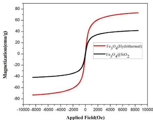
شکل 6. آنالیز VSM نانو ذرات \text{Fe}_3\text{O}_4 و هسته-پوسته \text{Fe}_3\text{O}_4@SiO_2 .
