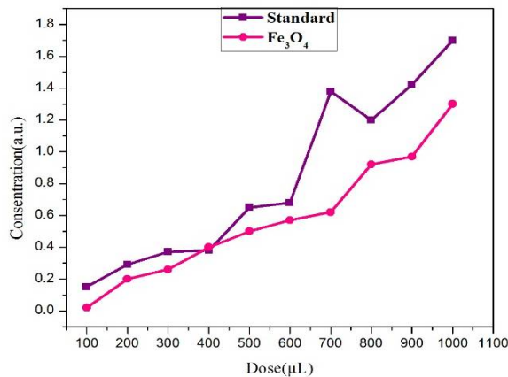
شکل 14. منحنی استاندارد دیازینون در مقایسه با Fe_3O_4 .
