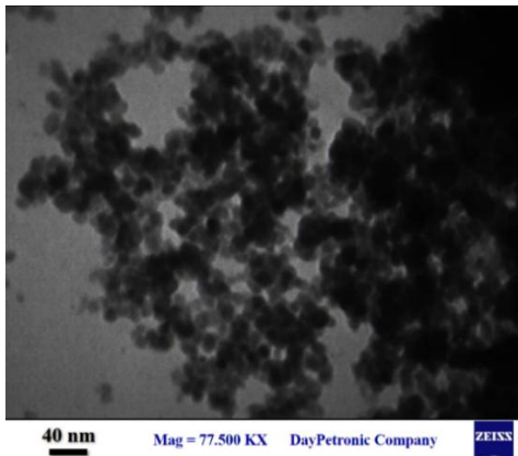
شکل 9. تصویر TEM نانوذرات Fe_3O_4@SiO_2 .
