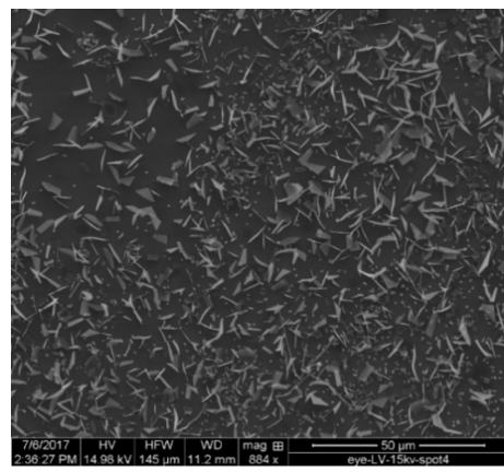
شکل 1. الف: تصویر شماتیک سیستم CVD. مکان زیرلایه و پیش ماده‌ها. تصاویر FESEM نانوپوسه‌های عمودی MoS 2 رشد یافته روی زیرلایه SiO 2 /Si به روش Sliding-CVD. ب: مراحل اولیه رشد ج: رشد نانوپوسه‌های عمودی.
