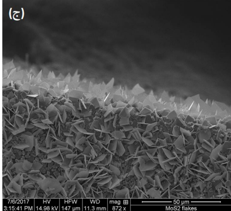
شکل 2. تصاویر FESEM اثر افزایش سرعت فوق اشباع بر رشد و تراکم نانوپوسه‌های عمودی MoS 2 رشد یافته روی زیرلایه SiO 2 /Si با جریان گاز آرگون 300 sccm به روش Sliding CVD الف: رشد پوسه‌های افقی در مراحل اولیه. ب: رشد نانوپوسه‌های عمودی بر روی نانورقه‌های افقی. ج: تصویر پوسه‌ها در لبه زیرلایه که نزدیک به منبع است.
