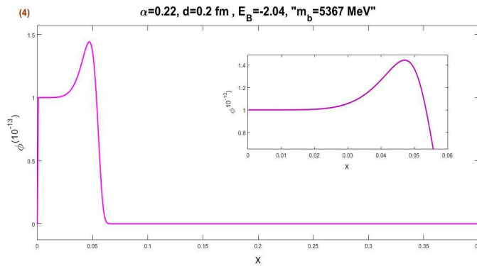
شکل 4. تابع موج \bar{b}bss برای d = 0.2\text{fm}, \alpha = 0.22, m_b = 5367\text{MeV}
