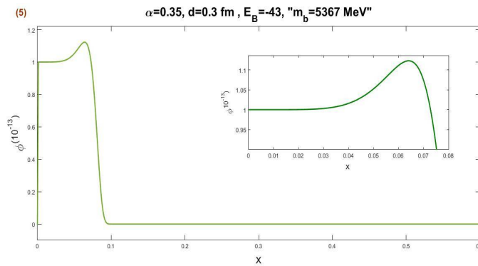
شکل 5. تابع موج \bar{b}bss برای d = 0.3\text{fm}, \alpha = 0.35, m_b = 5367\text{MeV}
