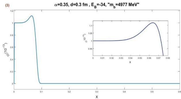
شکل 3. تابع موج \bar{b}bss برای d = 0.3\text{fm}, \alpha = 0.35, m_b = 4977\text{MeV}
