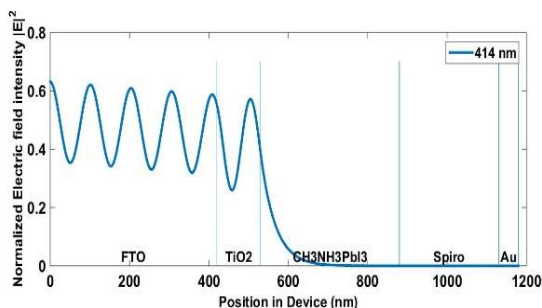
شکل 6. مجذور میدان الکتریکی سلول با \text{TiO}_2 به‌عنوان ETL
