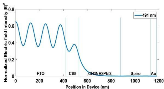
شکل 8. مجذور میدان الکتریکی سلول با \text{C}_{60} به عنوان ETL
