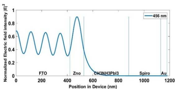
شکل 7. مجذور میدان الکتریکی سلول با ZnO به‌عنوان ETL
