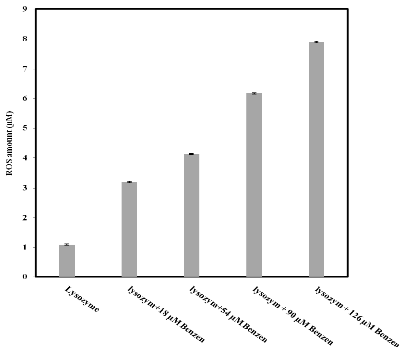
شکل ۵- نمودار مربوط به تولید گونه‌های فعال اکسیژن در حضور غلظت‌های مختلف بنزن. نمونه‌ها در در بافر کربنات ۱۰۰ میلی مولار با pH برابر ۹ حل شدند و داده‌ها در طول موج ۴۲۵ نانومتر جمع آوری شدند.
