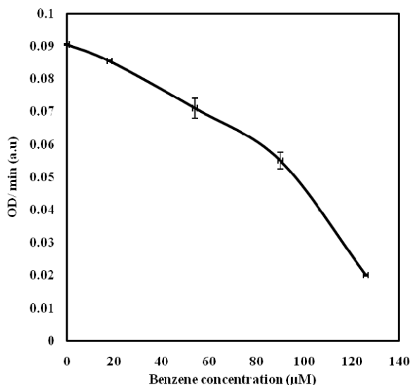
شکل ۴- طیف مربوط به فعالیت آنزیمی لیزوزیم در غیاب و حضور غلظت‌های مختلف بنزن. آنزیم با غلظت ۰/۱ میلی گرم بر میلی لیتر در بافر فسفات ۰/۱ مولار با pH برابر ۷ در دمای ۲۵ درجه سانتی گراد تهیه شد. جذب در طول موج ۴۵۰ نانومتر اندازه گیری شد. تولید گونه‌های فعال اکسیژن: شکل ۵ نمودار مربوط به تولید گونه‌های فعال اکسیژن در حضور بنزن است. نتایج فعال اکسیژن افزایش می‌یابد. نشان می‌دهد که با افزایش غلظت بنزن میزان گونه‌های
