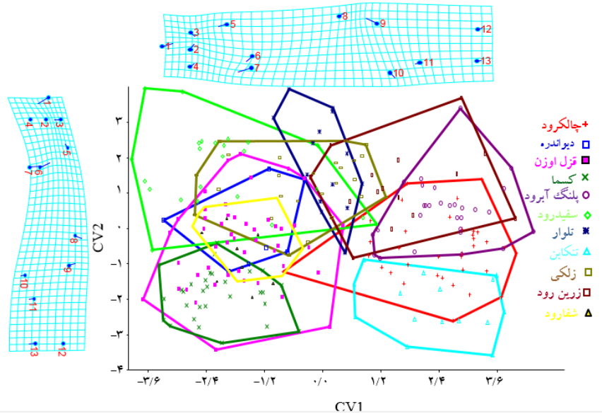
شکل ۴- نمودار تحلیل همبستگی کانونی (CVA) شکل بدن جمعیت‌های ماهی سفید رودخانه‌ای در بخش غربی حوضه خزر.
