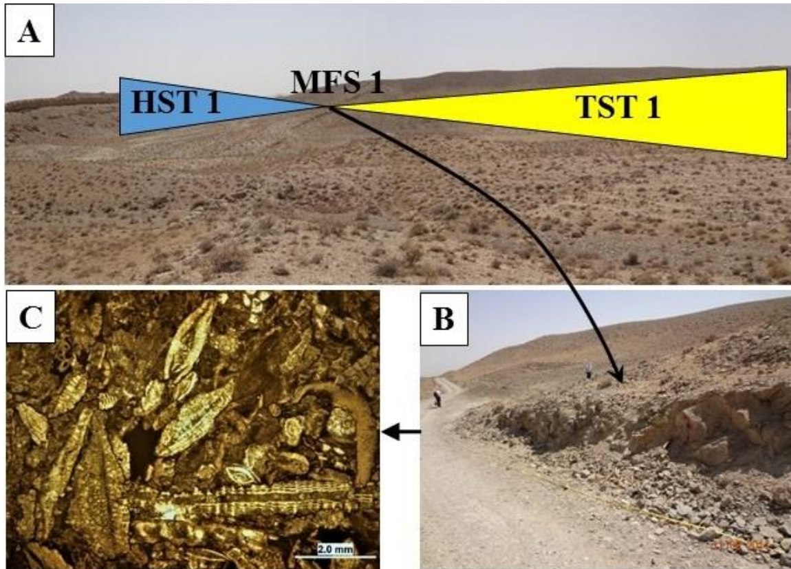
شکل ۹- A) عکس از سکناس اول و سیستم تراکت های TST 1، HST 1 و حداکثر پیشروی آب دریا (MFS 1)، B) عکس آهک های تشکیل شده طی حداکثر پیشروی آب دریا (MFS 1) C) عکس میکروسکوپی از مقطع نازک مربوط به آهک های تشکیل شده طی حداکثر پیشروی آب دریا (MFS 1).
