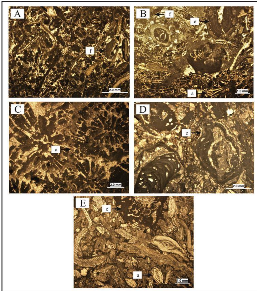
شکل ۵- میکروتافوفاسیس های سازند قم در ناحیه کهک، (A) میکروتافوفاسیس ۱، (F: خردشده)، (B) میکروتافوفاسیس ۲، (F: خردشده)، (E: قشرسازی، (A: ساییدگی، (C) میکروتافوفاسیس ۳، (A: ساییدگی، (D) میکروتافوفاسیس ۴، (E: قشرسازی، (E) میکروتافوفاسیس ۵، (A: ساییدگی، (E: قشرسازی.
